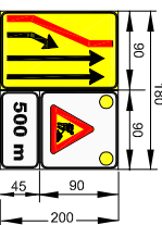
fig. II 399/a Art. 39 Presegnale di cantiere mobile (misura ridotta)
