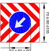
fig. II 389 Art. 38 Passaggio obbligatorio per veicoli operativi
