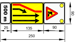
fig. II 399/a Art. 39 Presegnale di cantiere mobile (misura ridotta)
