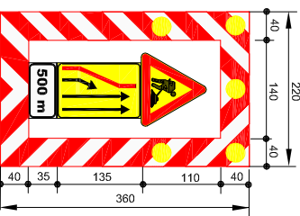
fig. II 400 Art. 39 Segnale mobile di preavviso
