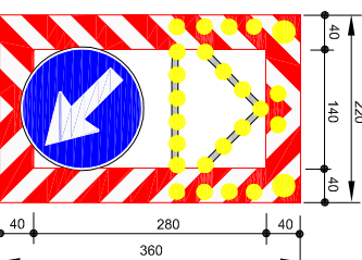
fig. II 401 Art. 39 Segnale mobile di protezione
