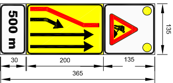
fig. II 399/a Art. 39 Presegnale di cantiere mobile
